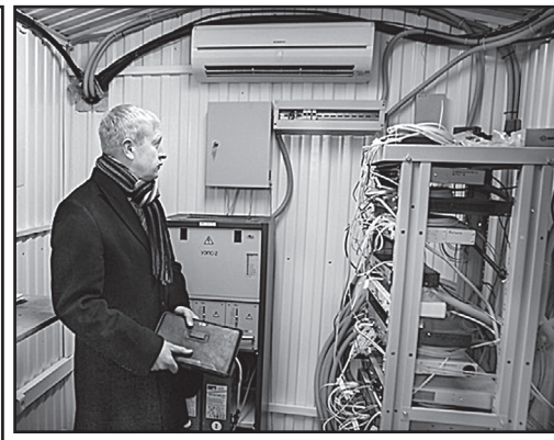
Оборудование, обеспечивающее работу точки Wi-Fi
