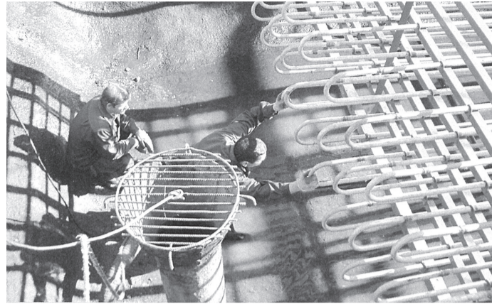
► Установка тепловых насосов на биологических очистных сооружениях г. Тобольска для обогрева производственных помещений, 2005 г. В качестве источника тепла используются сточные воды с температурой +15...+18°С
