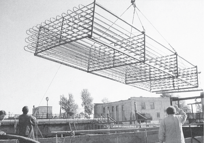
► В теплообменниках нагревается до температуры +15...+16°С чистая вода, которая подаётся к тепловым насосам по системе трубопроводов
