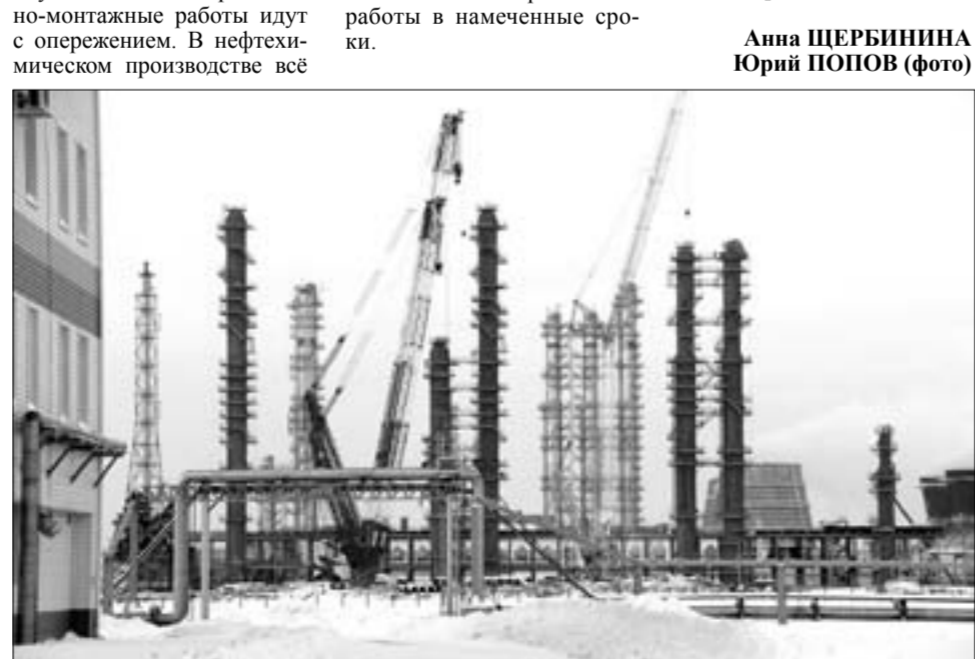
Газофракционирующая установка № 2
