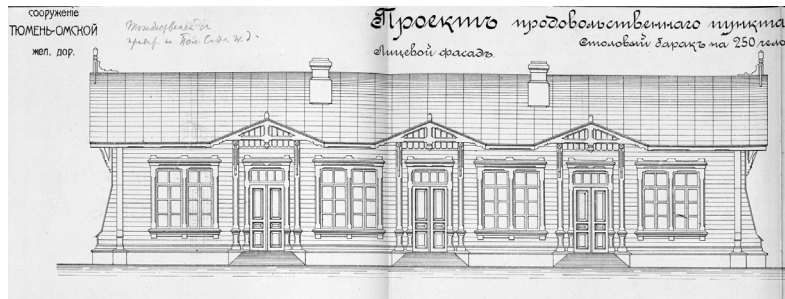
Проект столовой военно-продовольственного пункта.
