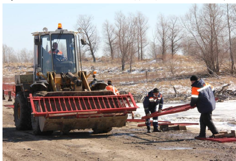
Защитные устройства грузят на спецтехнику // Фото автора
